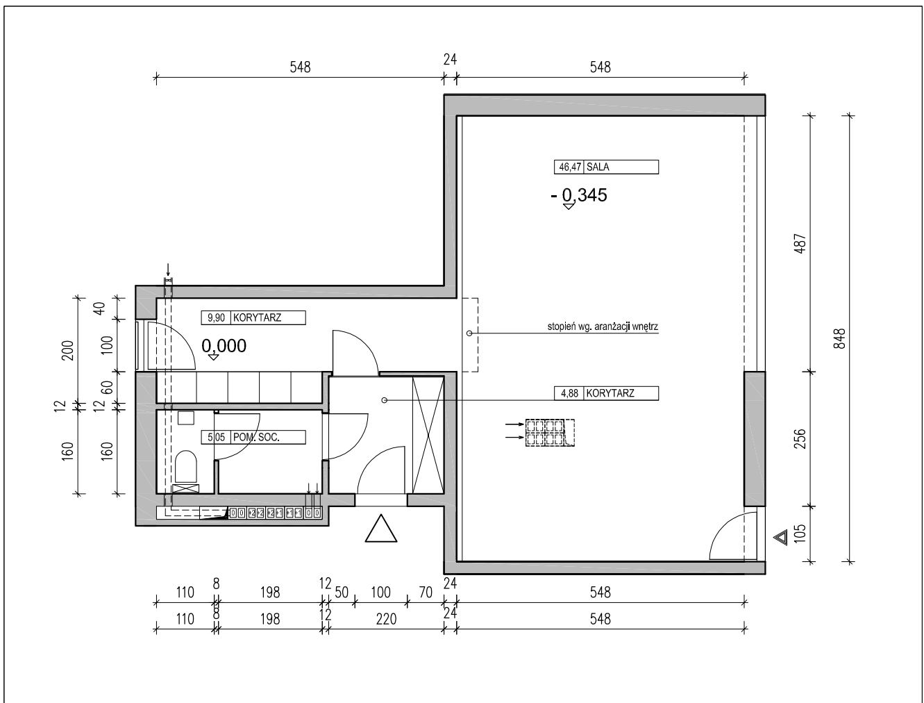
RZUT 1:100
