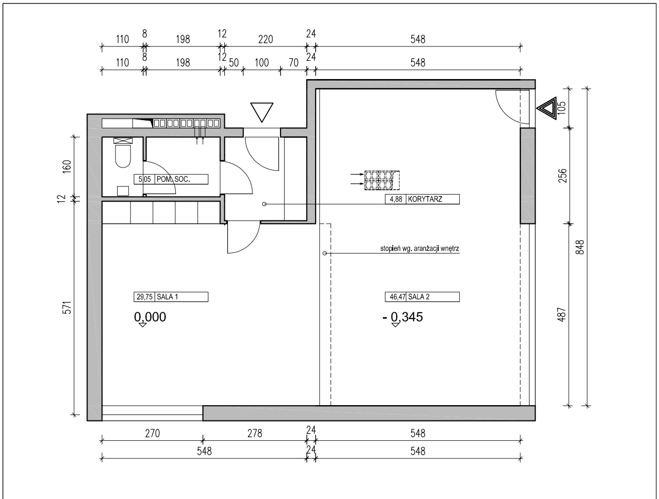
RZUT 1:100
